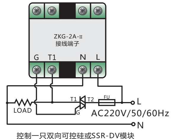
ZKG-2A-II调整器接线图
